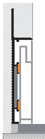
Instalación con cierre total
