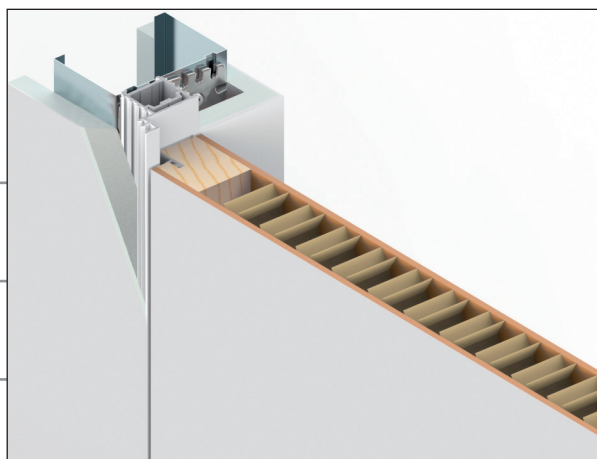
Aplicación para cartón yeso
