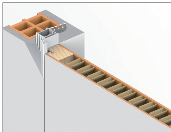
Aplicación para revoque
