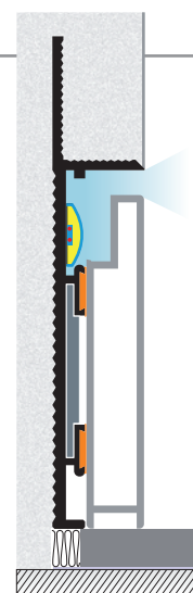
Instalación con retroiluminación LED
