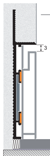
Instalación con ranura de 3mm
